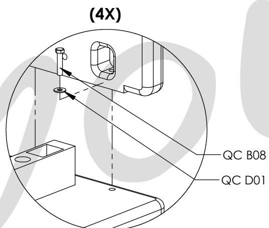
DÉTAIL B
