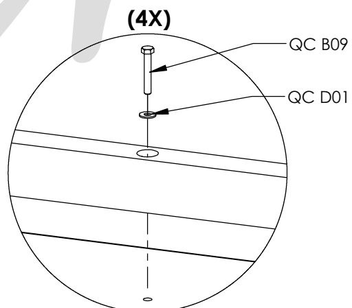
DÉTAIL A
